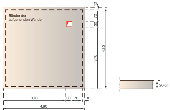
Abb. 46 – Lage des nachträglich hinzugefügten Durchbruchs in der Platte
