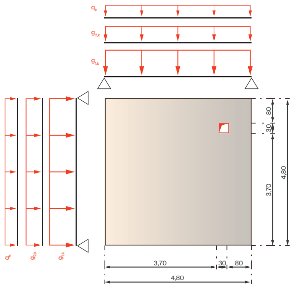
Abb. 47 – System und Lasten
