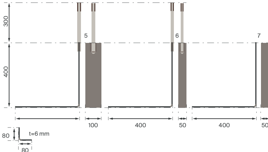
Abb. 40 – Stahlwinkel für Stahllaschen
