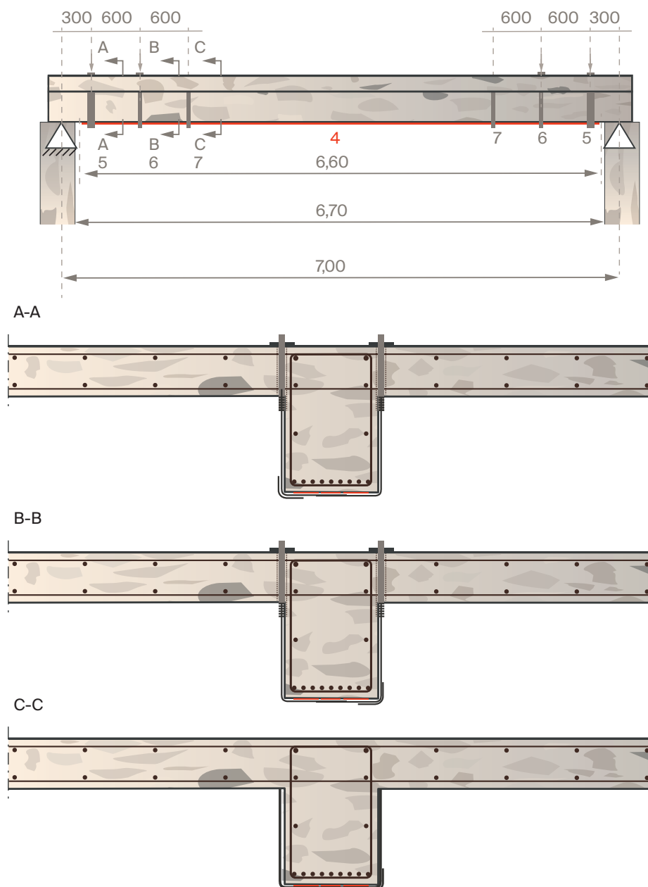
Abb. 39 – Anordnung der Klebelamellen
