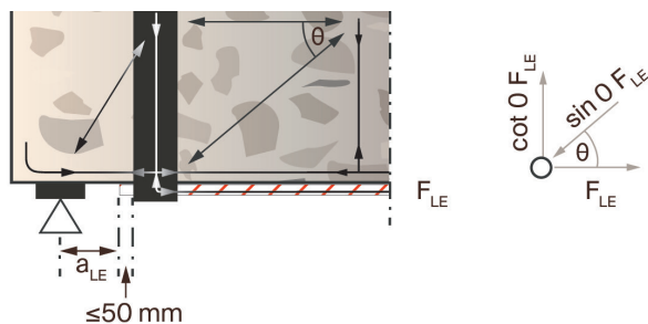
Abb. 35 – Bügelkraft aufgrund der Zugkraft der Biegeverstärkung (Grundlage: DAfStb Heft 595, Bild H.26)
