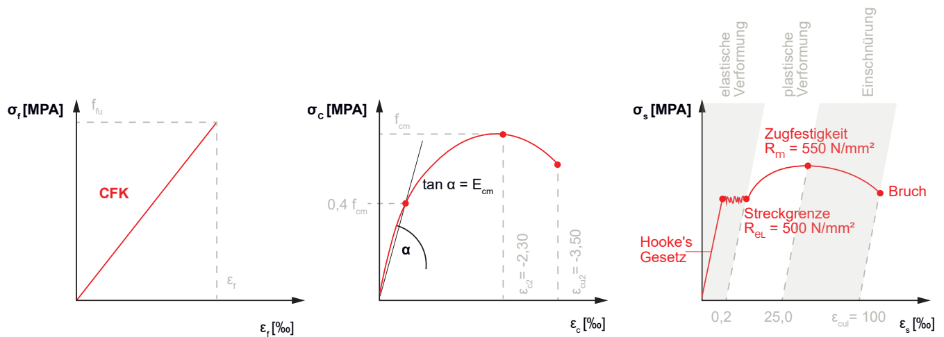
Abb. 2 – Spannungs-Dehnungs-Diagramme - links: CFK, Mitte: Beton, rechts: Betonstahl
