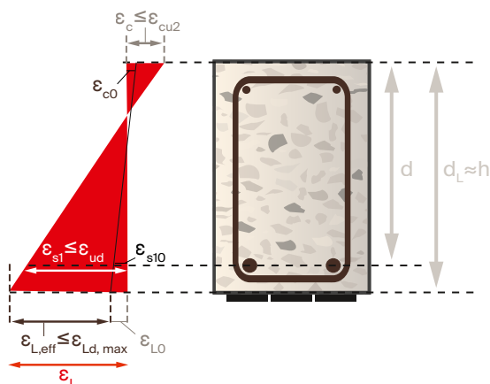
Abb. 14 – Dehnungsverteilung in einem gerissenen Querschnitt unter Berücksichtigung der Vordehnung der Stahlbewehrung
