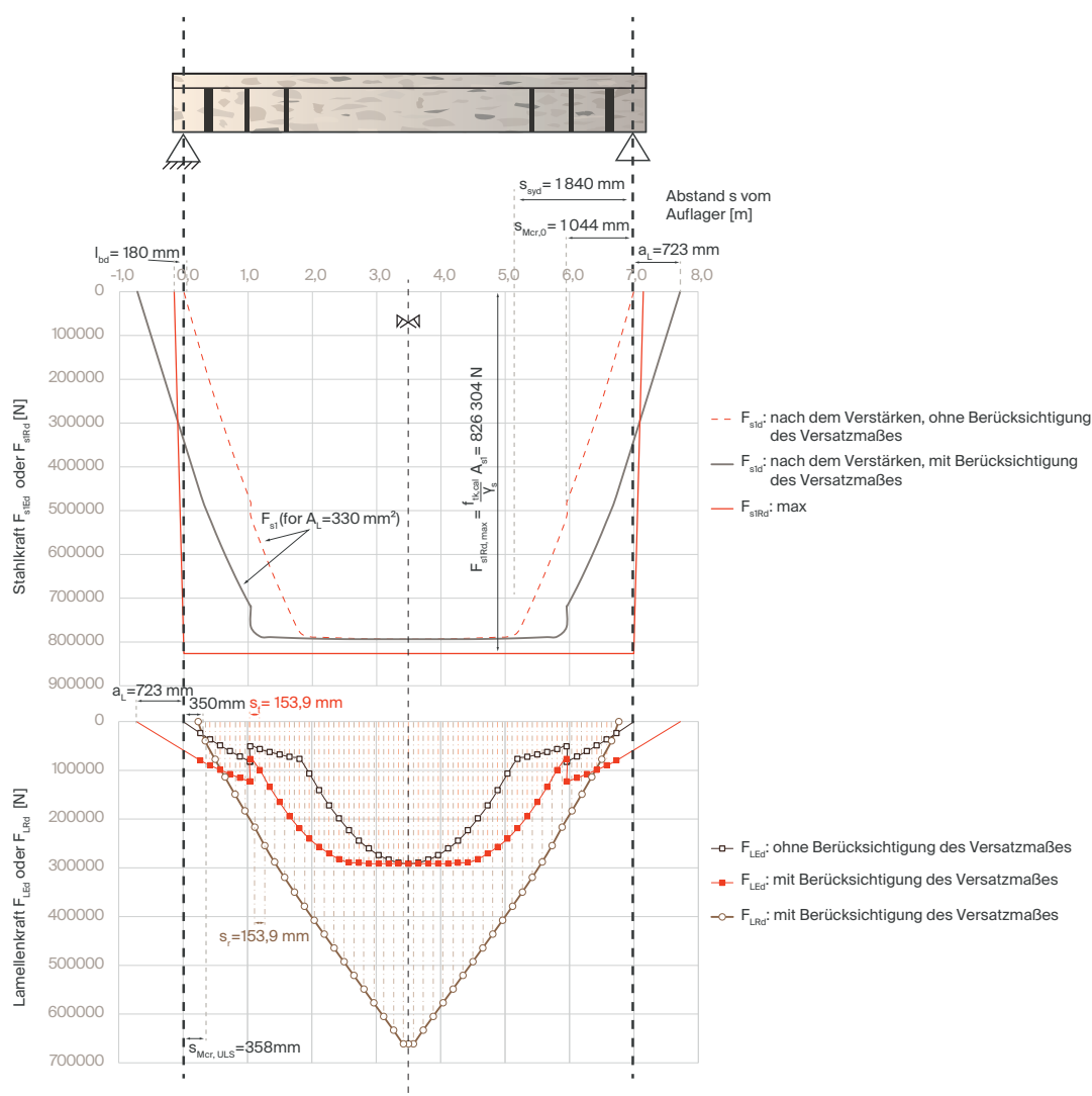
Abb. 38 – Grafische Darstellung der verschobenen Zugkraftlinie und dem Widerstand der Zugkraftlinie für die Lamellen
