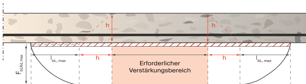
Abb. 51 – Örtliche Verstärkung mit CFK-Lamellen nach Bild H12 des DAfStb Heftes 595
