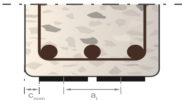
Abb. 50 – Erläuterungen zu den Lamellenabständen in Abbildung H22 des DAfStb-Heftes 595 2
