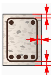
Abb. 25 – Betondeckung
