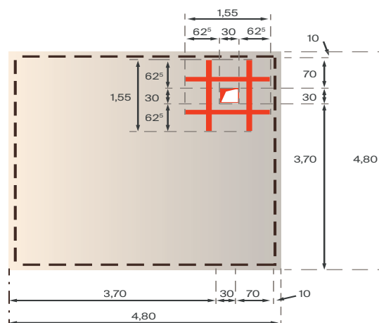
Abb. 52 – Identische Anordnung der aufgeklebten CFK-Lamellen an der Ober- und Unterseite der Platte zur lokalen Verstärkung (Grundriss)
