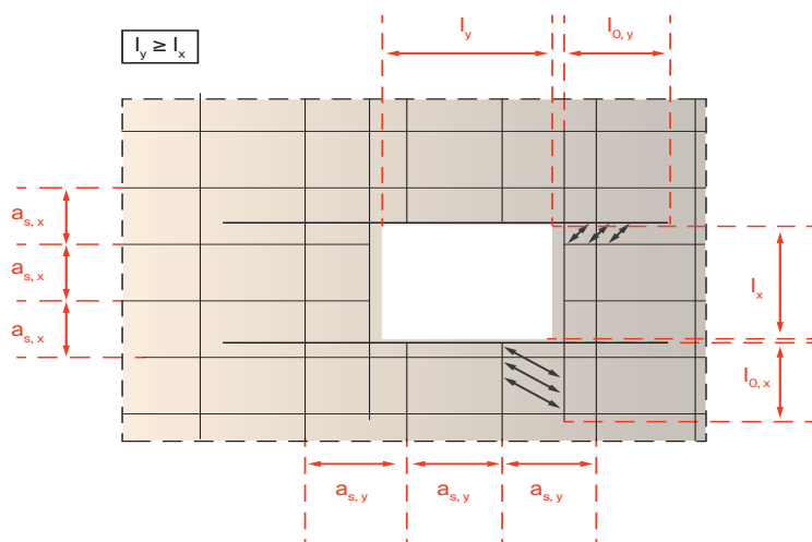
Abb. 49 – Bezeichnungen am Durchbruch
