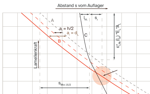
Abb. 44 – Verschobene Lamellenzugkraftlinie an der Stelle der Endverankerung ( s_{\text{McT,ULS}} )
