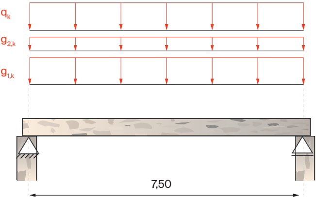
Abb. 42 – Einwirkende Streckenlasten
