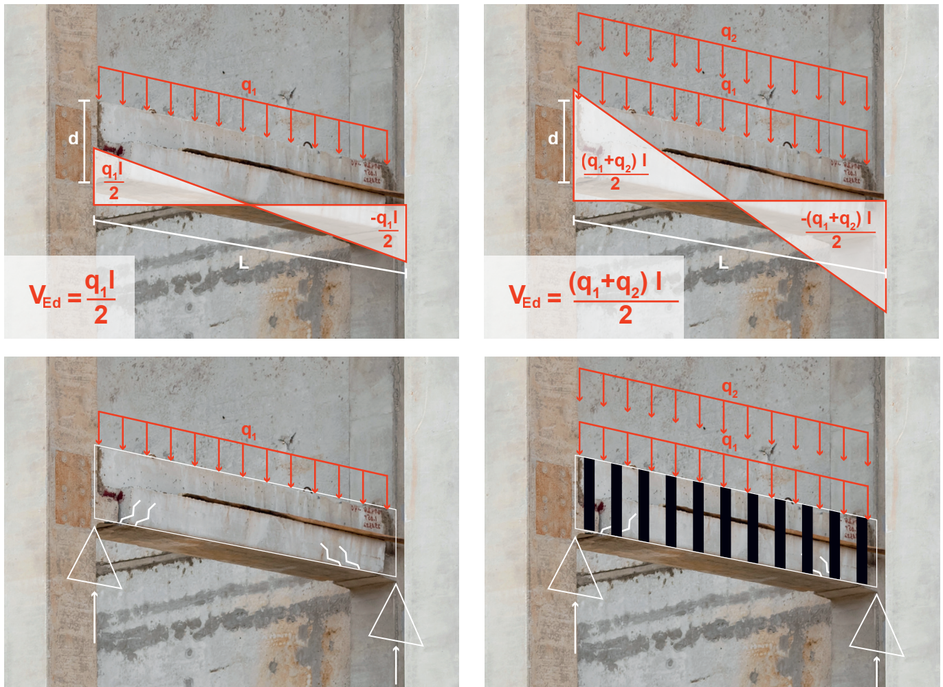
Abb. 5 – links: unverstärkter Träger, rechts: mit Querkraftverstärkung
