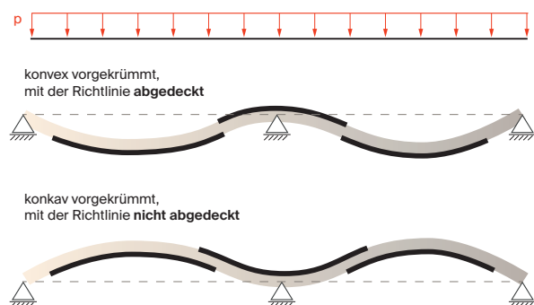
Abb. 13 – Bei aufgeklebten CFK-Lamellen und CF-Gelegen zulässige und nicht zulässige Richtung der Vorkrümmung
