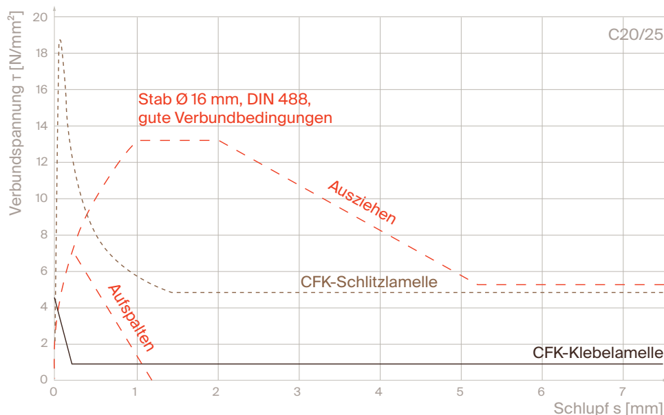
Abb. 10 – Spannungs-Schlupf-Verhältnis von geklebter Bewehrung und eingebetteter Stahlbewehrung
