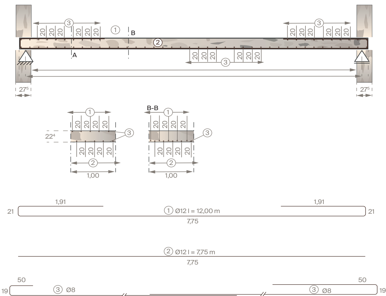
Abb. 41 – System, Querschnitt und Bewehrungsanordnung
