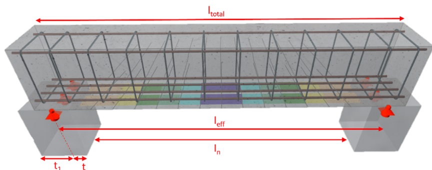
Abb.22 - Definition der Längen
