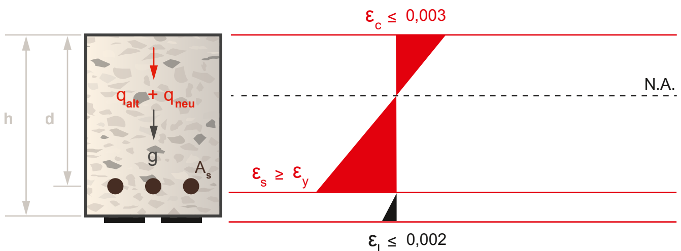
Abb. 3 - Verteilung der Dehnungen in Beton, Bewehrungsstahl und CFK
