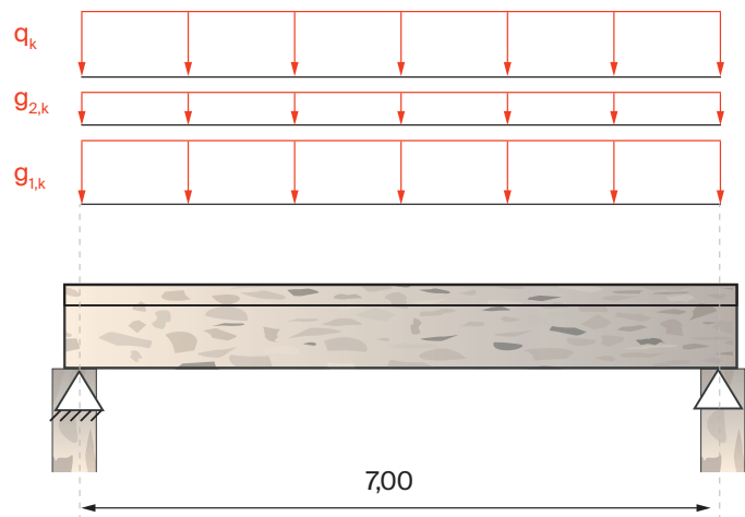
Abb. 25 – Einwirkende Streckenlasten
