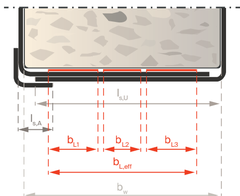
Abb. 37 – Anordnung von CFK-Lamellen und einem geklebten Bügel aus Stahlwinkeln an der Unterseite des Stegs
