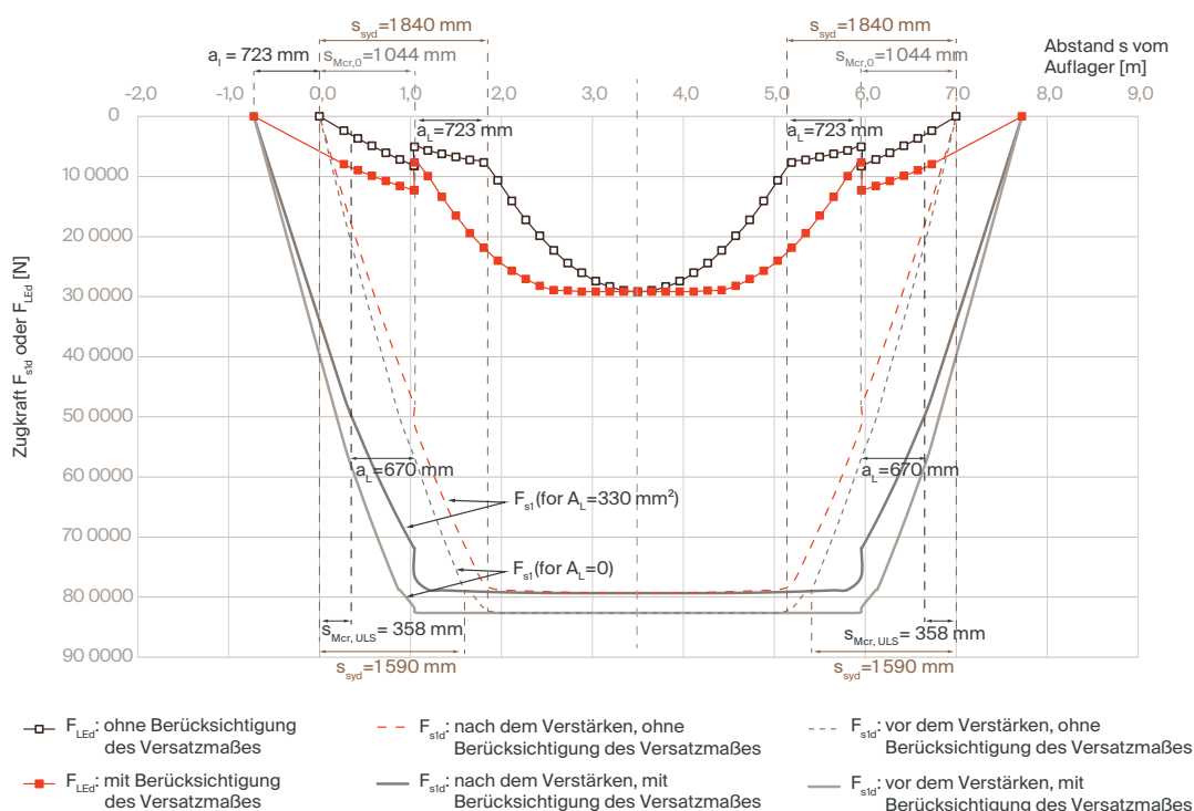
Abb. 36 – Stahl- und Lamellenzugkräfte im GZT
