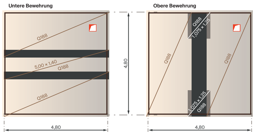
Abb. 48 – Bewehrungsanordnung
