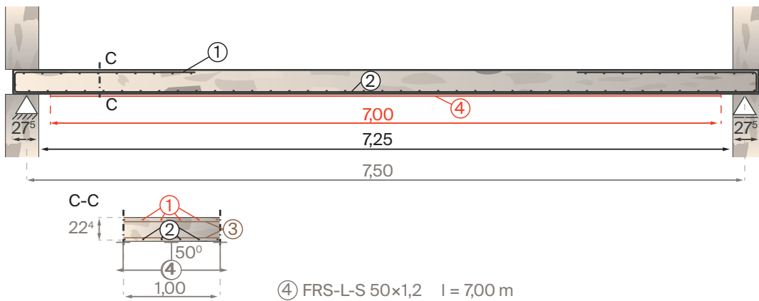
Abb. 45 – Anordnung der CFK-Lamellen
