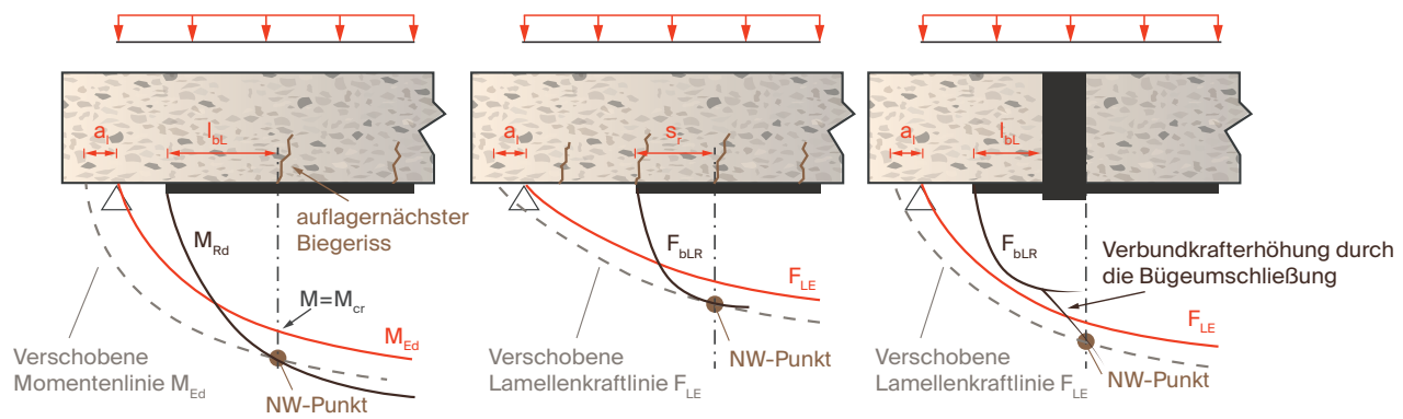
Abb. 15 – Konzepte für den Nachweis der Endverankerung nach der Richtlinie
