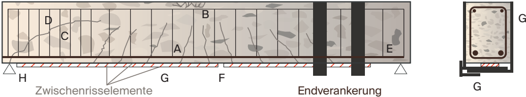
Abb. 8 – Versagensarten bei Trägern, die mit geklebter Bewehrung verstärkt sind
