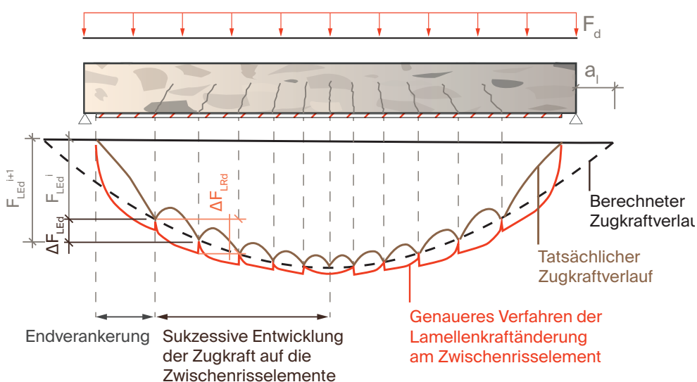
Abb. 11 – Genaueres Verfahren der Lamellenkraftdifferenz am Zwischenrisselement nach DAfStb
