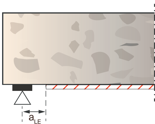
Abb.43 – Abstand a_{LE} des Lamellenendes vom rechnerischen Mittelpunkt
