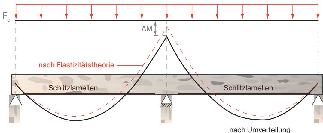
Abb. 7 – Kombination aus Umverteilung des Stützmoments und Verstärkung in den Bereichen der Feldmomente
