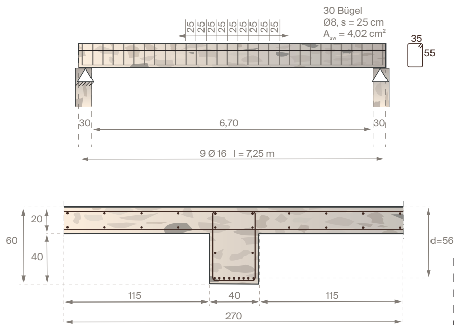
Abb.33 – System, Querschnitt und Bewehrungsanordnung
