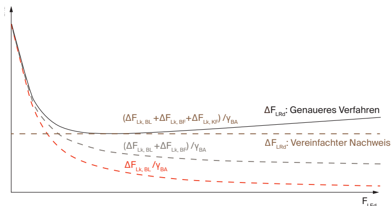
Abb. 12 – Aufnehmbare Lamellenkraftänderung am Zwischenrisselement
