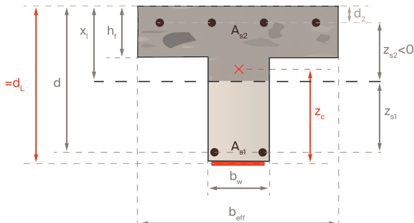
Abb. 34 – Bezeichnungen T-Querschnitt, Lage der Nulllinie im ungerissenen Zustand (nach Fingerloos/Hegger/ Zilch: Eurocode 2 für Deutschland und ergänzt)
