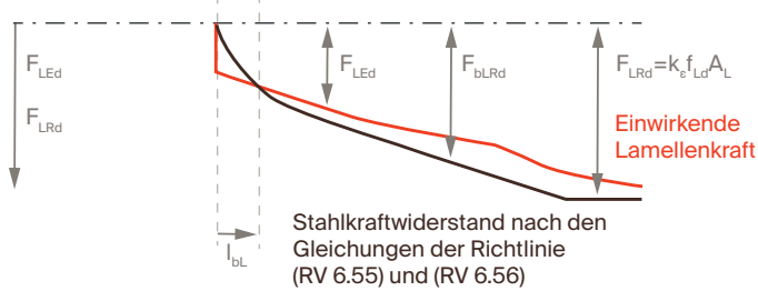
Abb. 16 - Verankerungsnachweis der in Schlitz verklebten CFK-Lamellen
